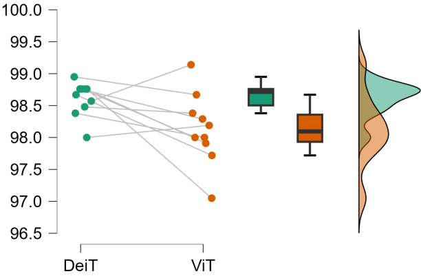
DeiT - ViT
