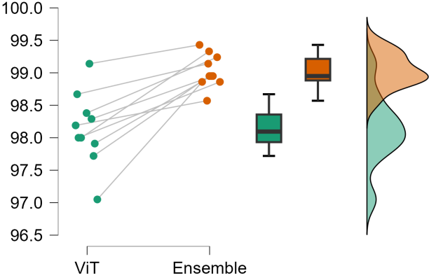
ViT - Ensemble
