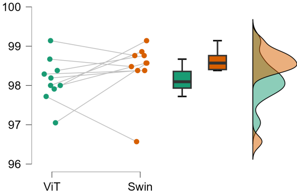
ViT - Swin
